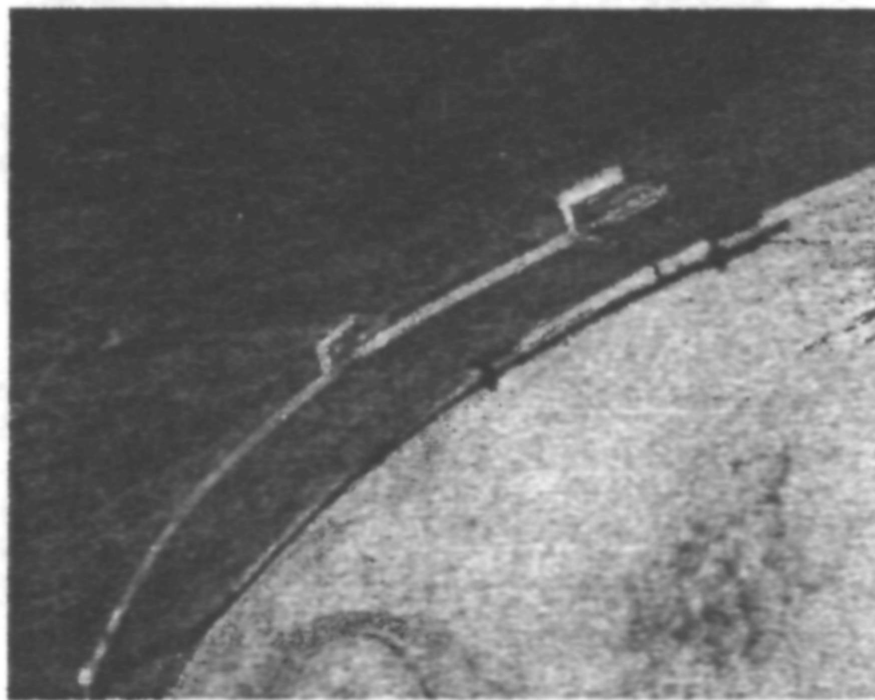
Рисунок А.5. Датчики контроля раскрытия трещин: а – механический датчик контроля раскрытия трещин (диапазон измерения 4 мм, шаг 0,2 мм, разрешение до 0,02 мм); б – шаблон для оценки раскрытия трещин; в – оптоволоконный датчик на трещине в своде Благовещенского собора Московского Кремля (база измерения 250 мм, разрешение 0,002 мм, относительная деформация 8 \cdot 10^{-6} )
