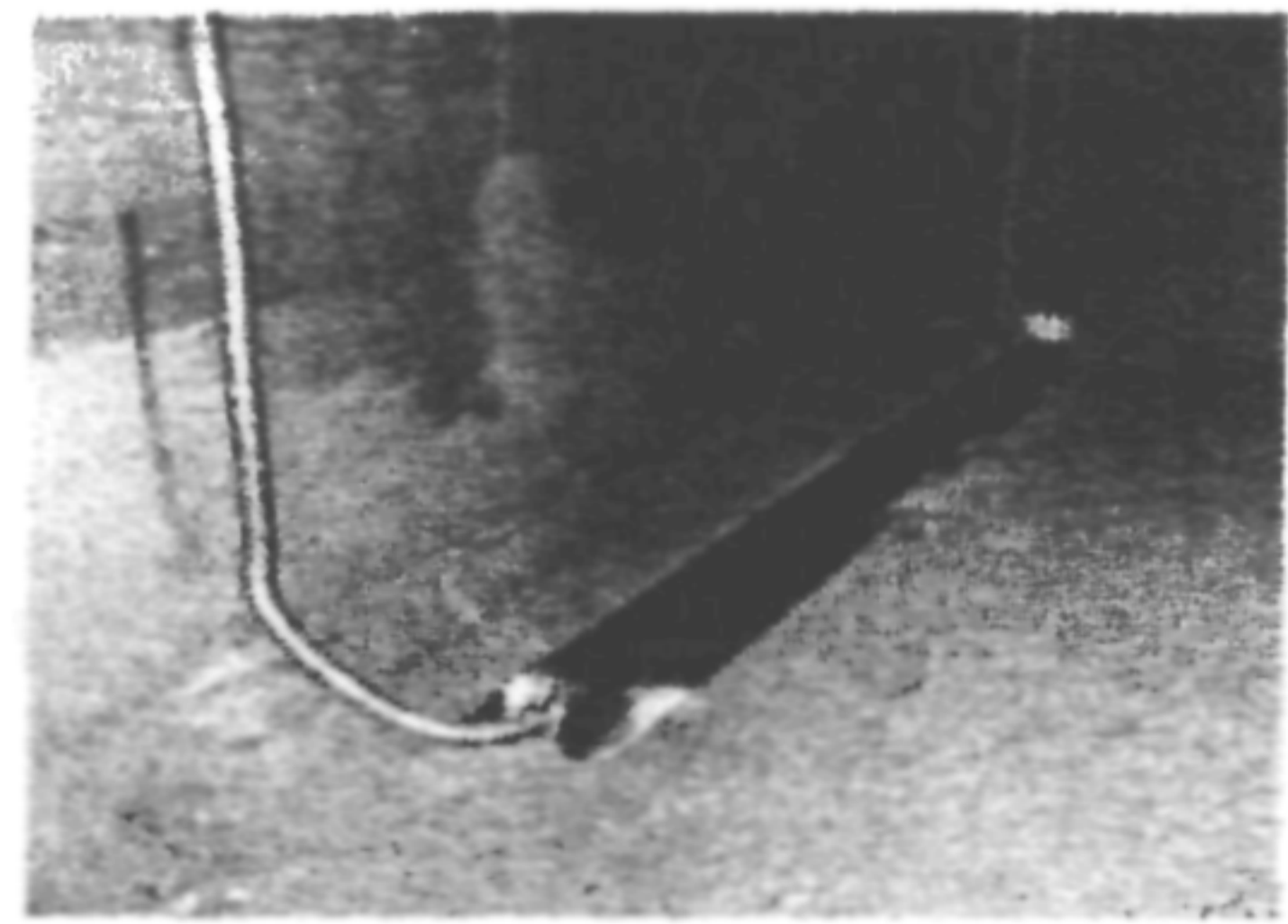
Установка сенсора с термопарой на опоре моста
